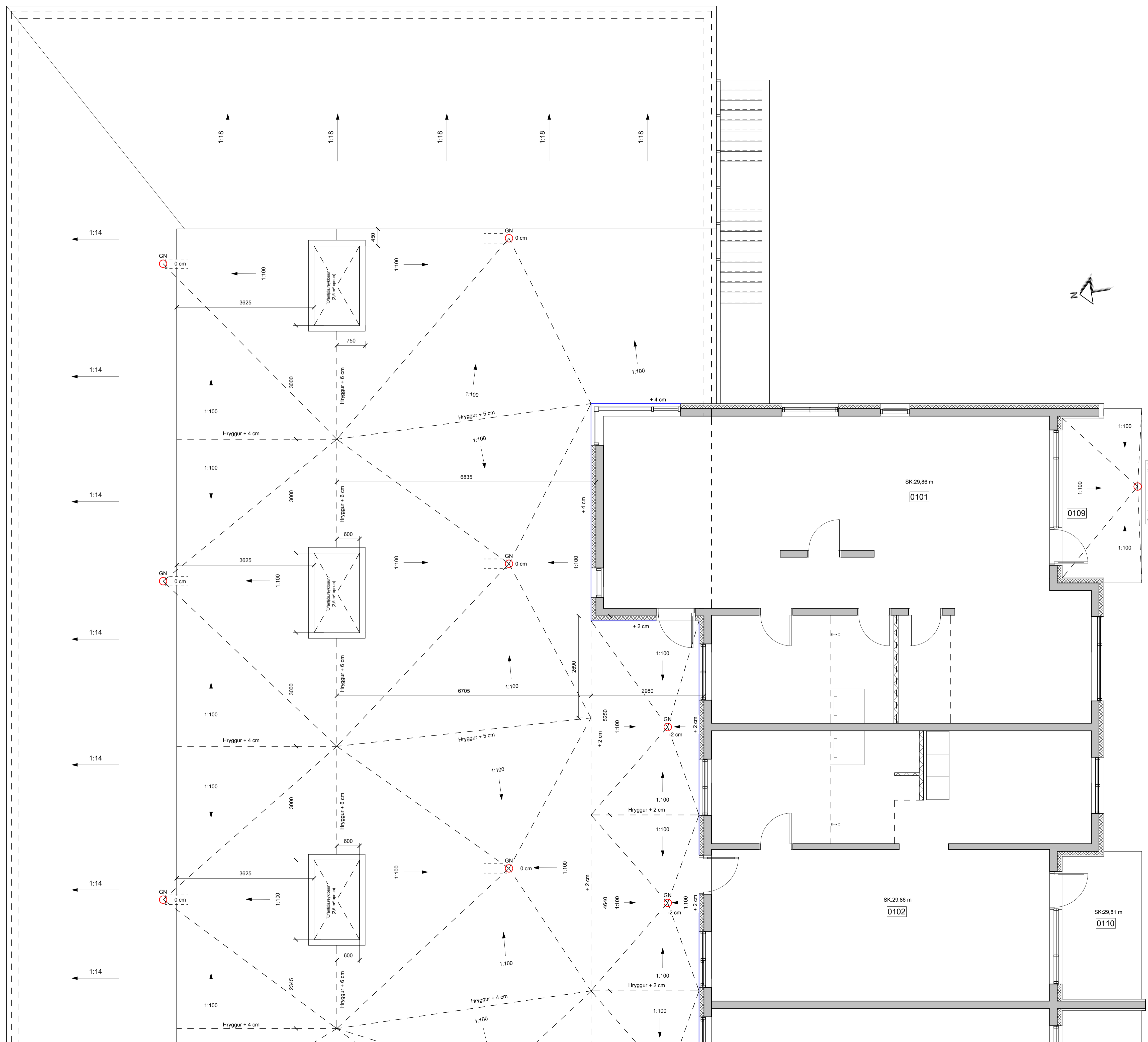
1. HÆÐ - VATNSHALLAPLAN - A mkv: 1 : 50
