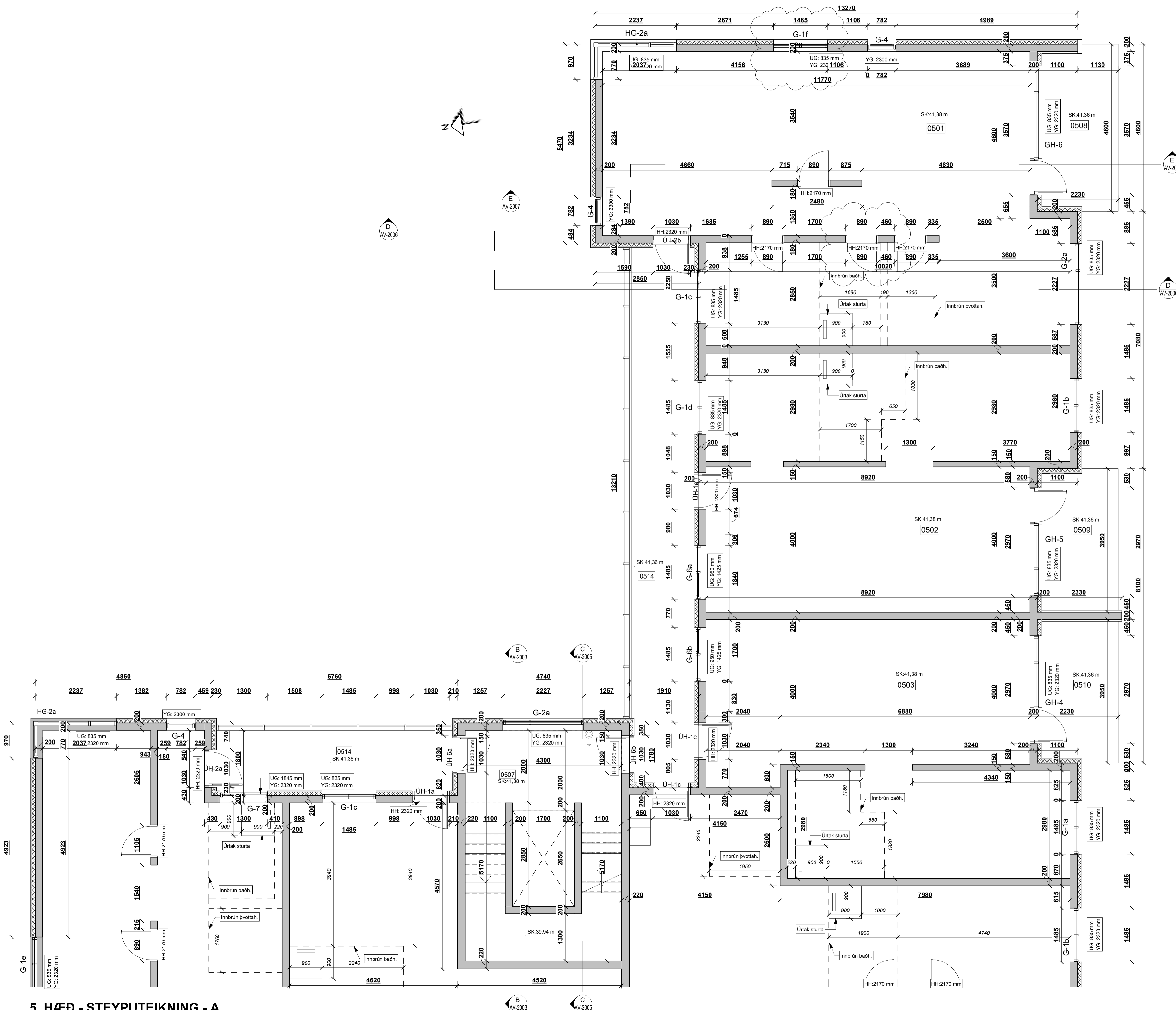
5. HÆÐ - STEYPU TEIKNING - A mkv: 1: 50
