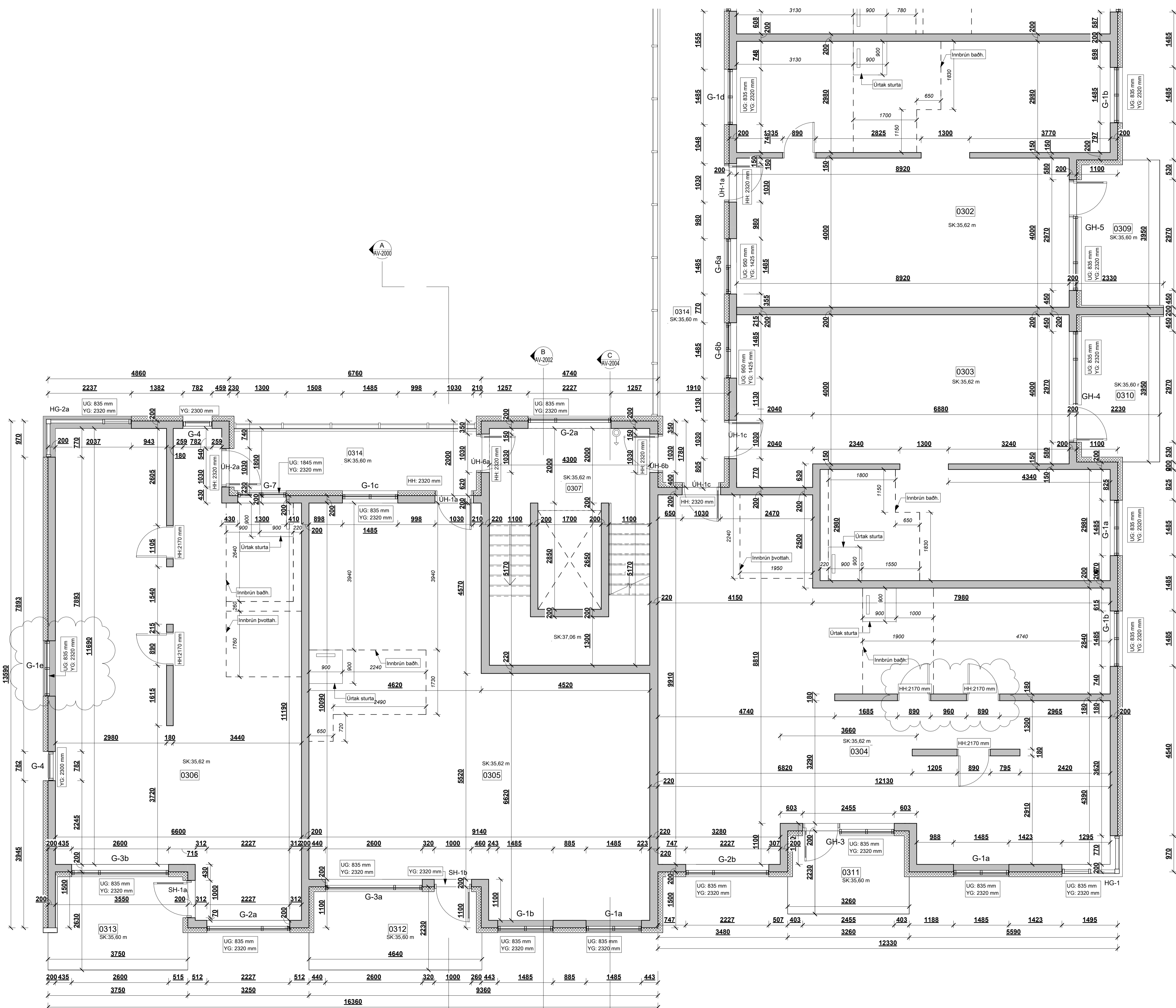
3. HÆÐ - STEYPU TEIKNING - B mkv: 1 : 50
