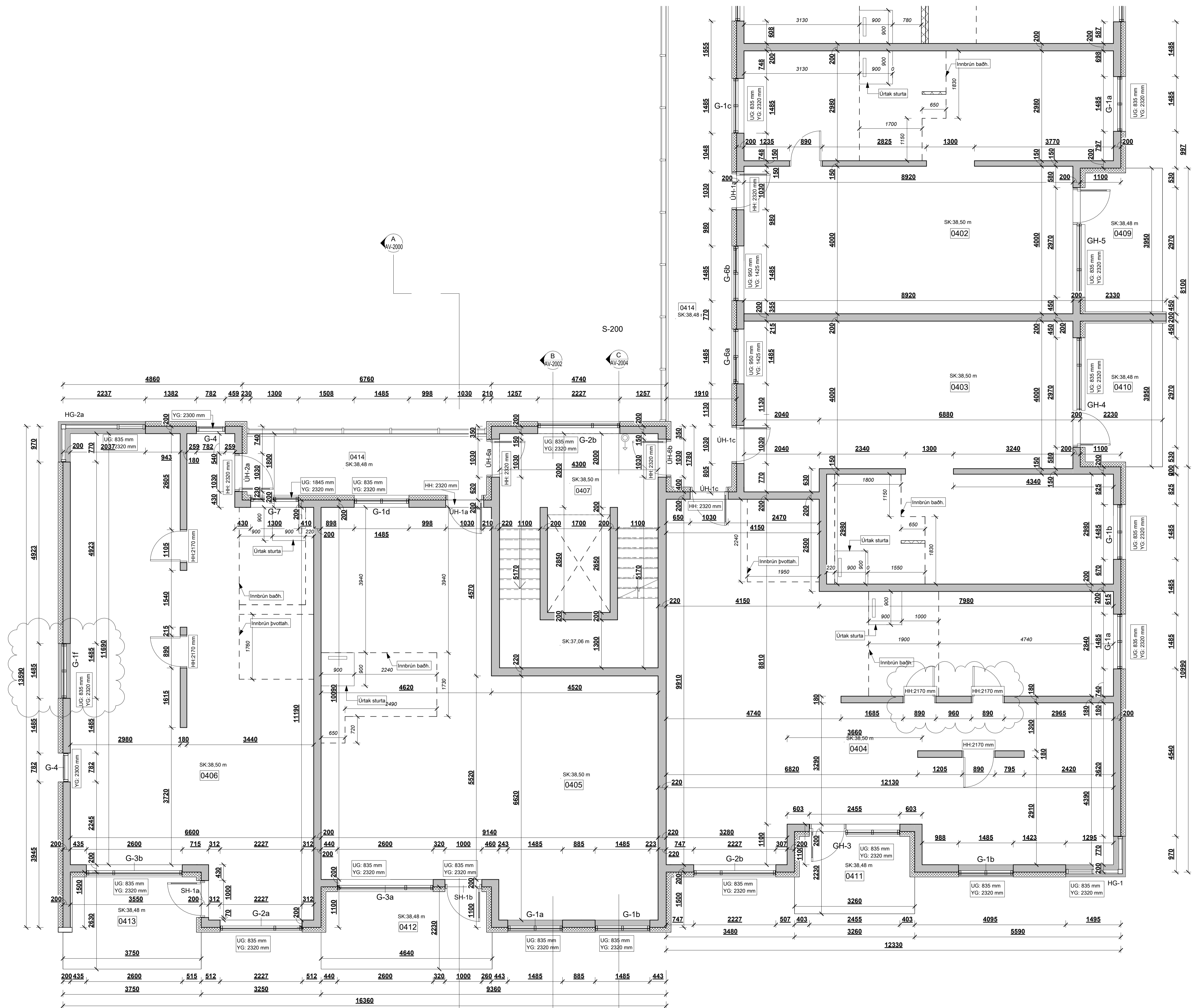
4. HÆÐ - STEYPU TEIKNING - B mkv: 1 : 50
