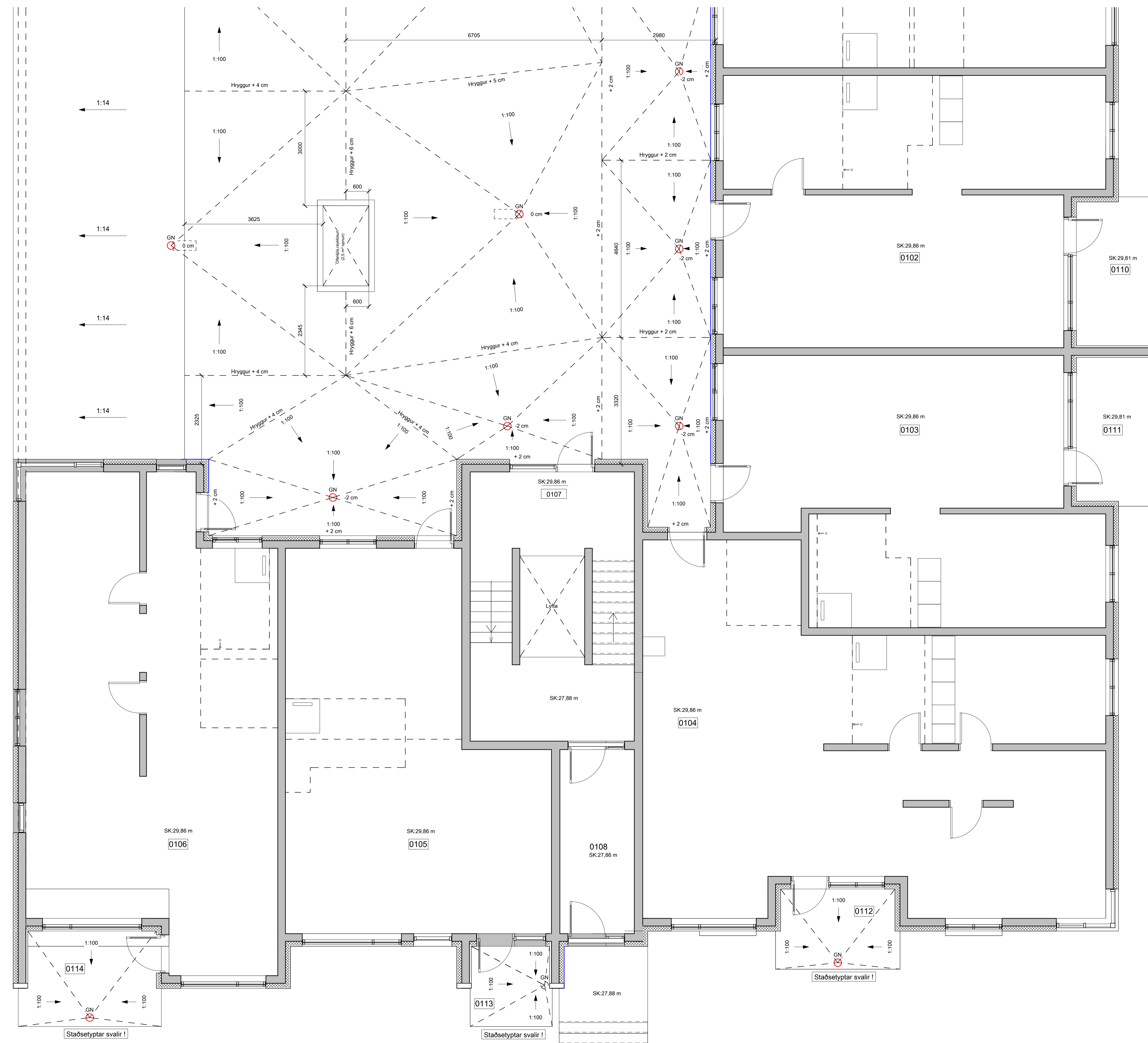
1. HÆÐ - VATNSHALLAPLAN - B mkv: 1 : 50
