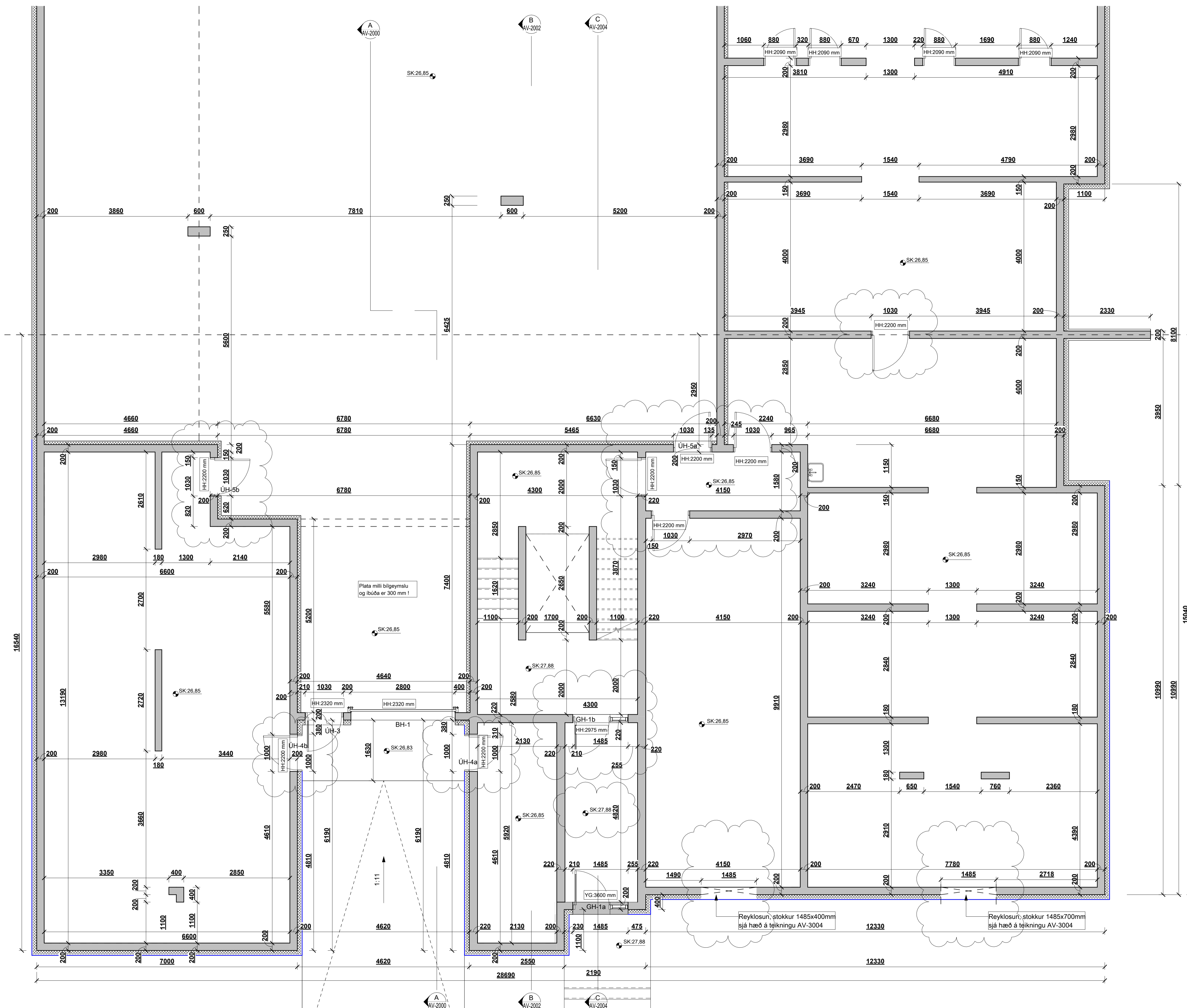
KJALLARA STEYPU TEIKNING - B mkv: 1 : 50
