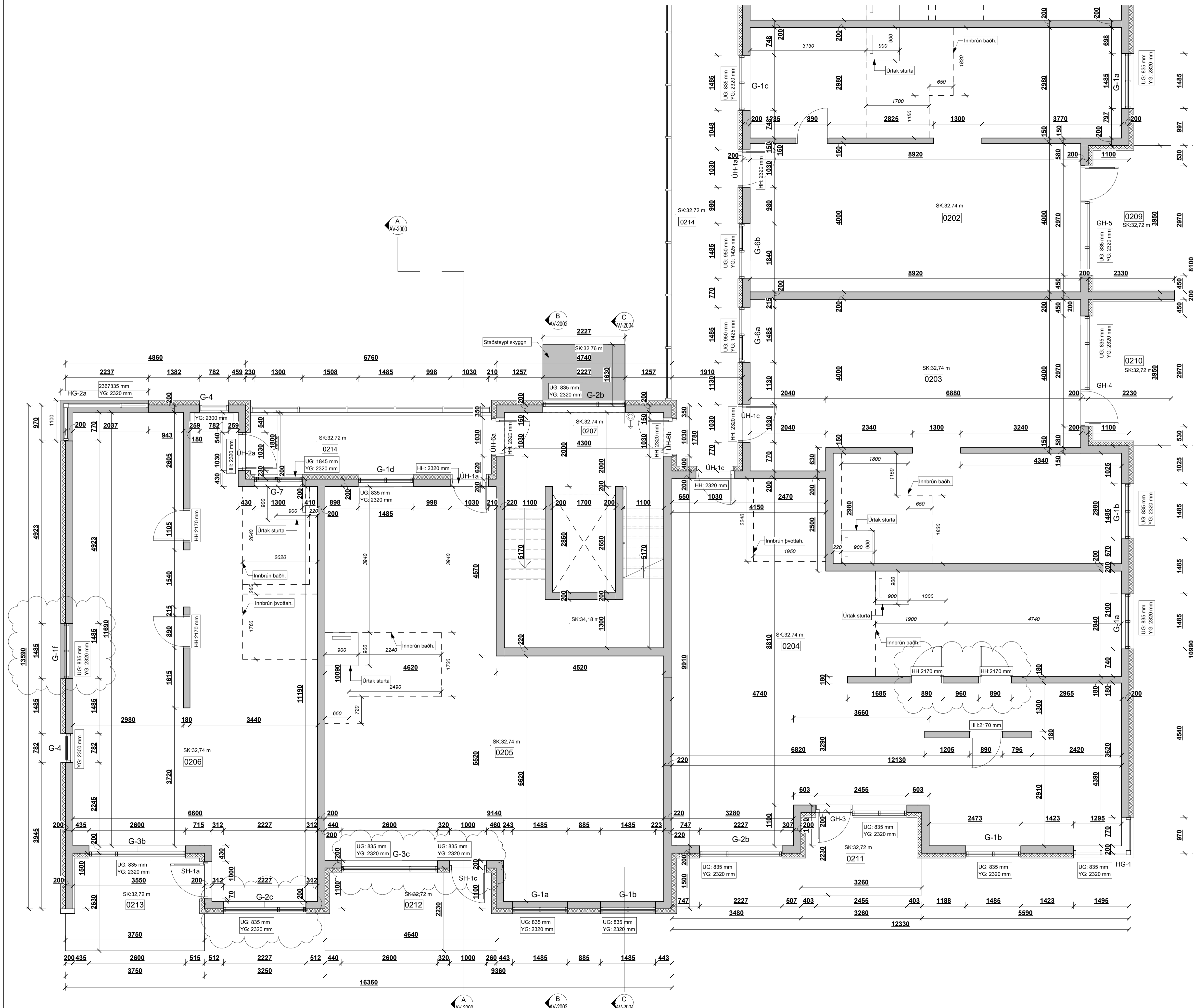
2. HÆÐ - STEYPU TEIKNING - B mkv: 1 : 50
