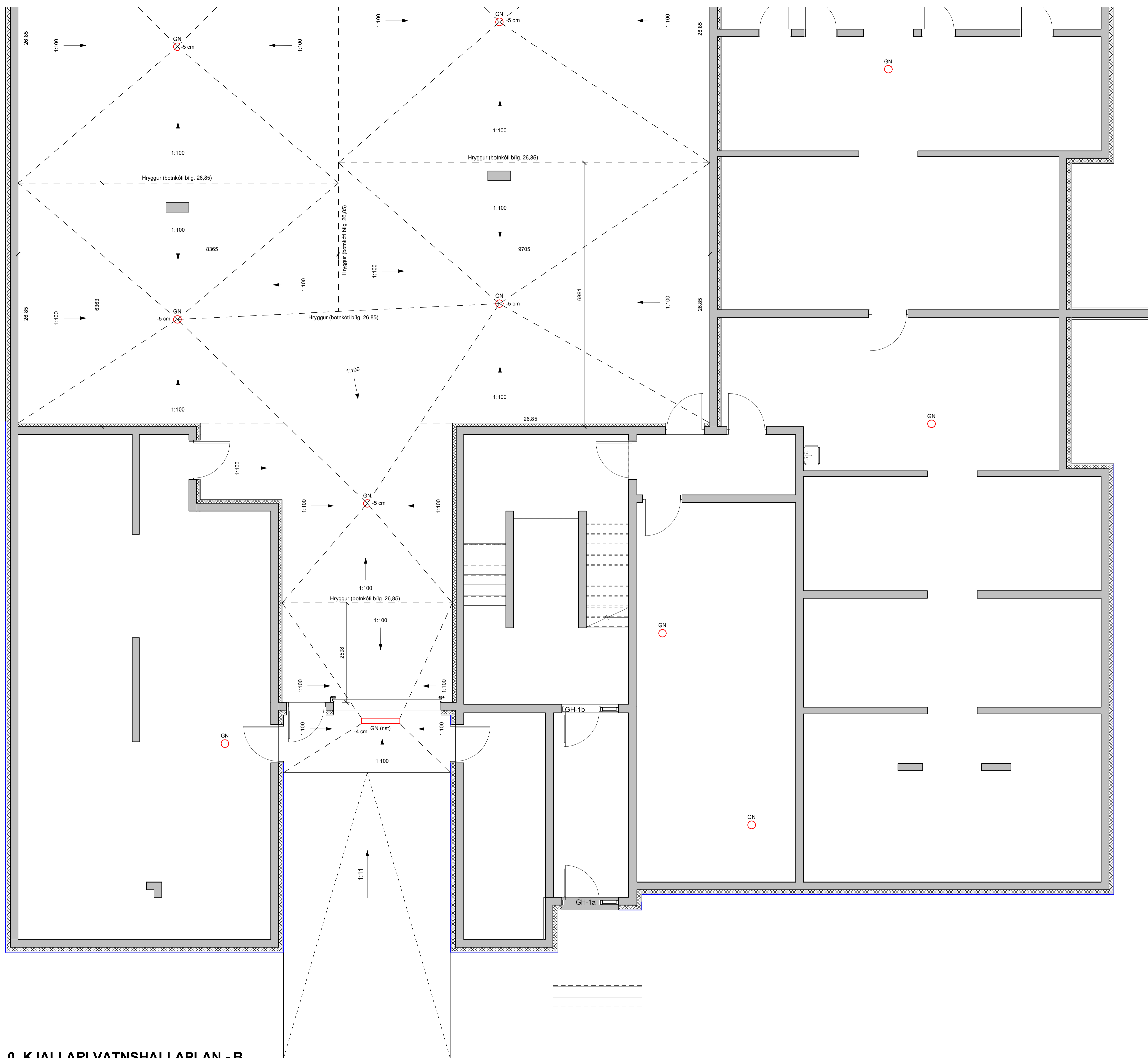
0. KJALLARI VATNSHALLAPLAN - B mkv: 1 : 50
