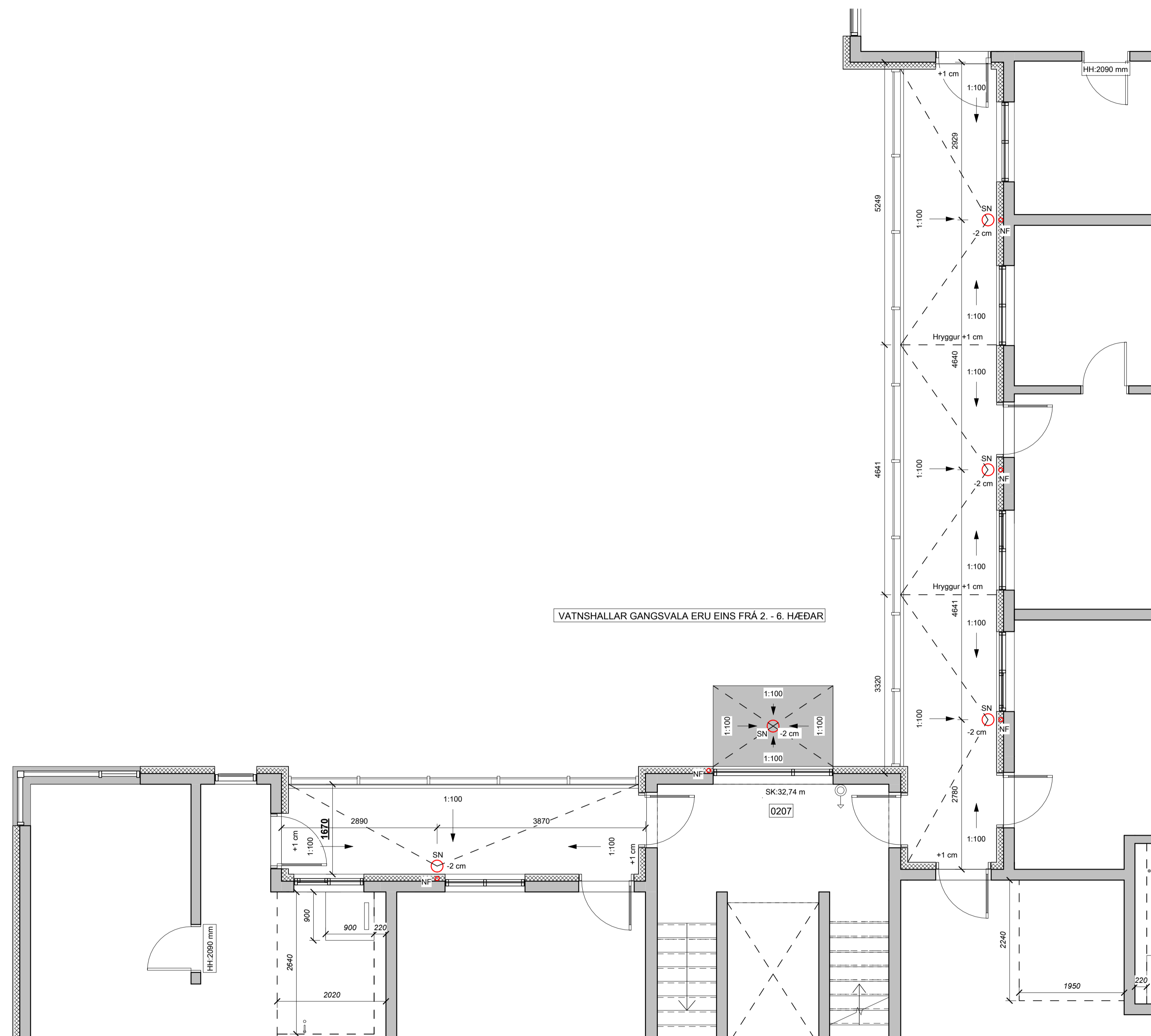
2.- 6. HÆÐ - VATNSHALLAPLAN mkv: 1 : 50
