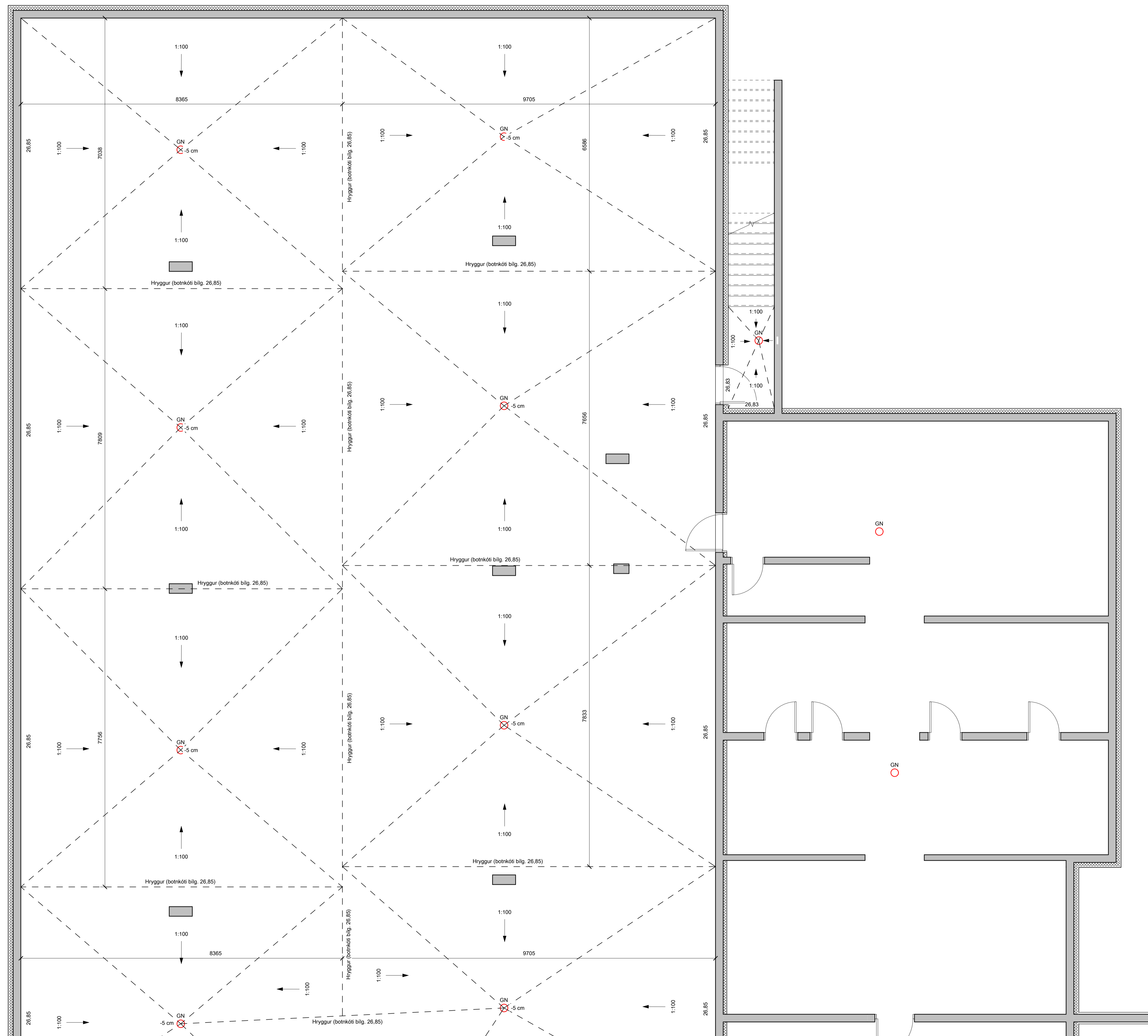
0. KJALLARI VATNSHALLAPLAN - A mkv: 1 : 50
